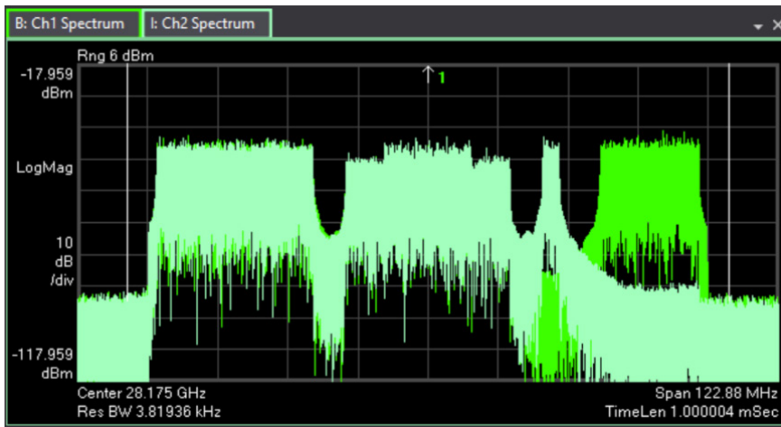
Figure 3a. 5G NR 28 GHz MIMO spectrum
